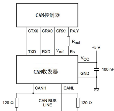
图 7 汽车应用瞬变测试电路
