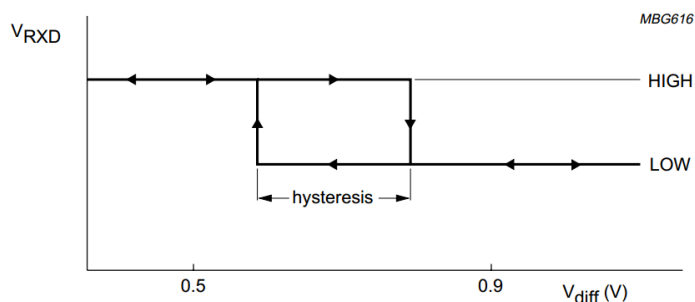
图 4 迟滞
