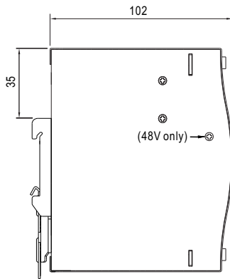
侧面图
