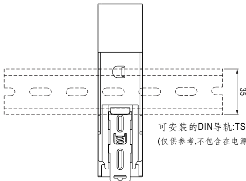
背面图
